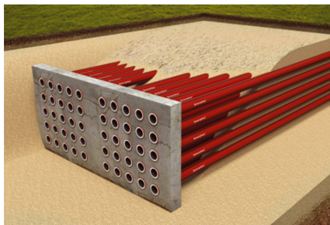
Рис. 13. Вариант применения труб ПротекторФлекс® БК для устройства блочной канализации
