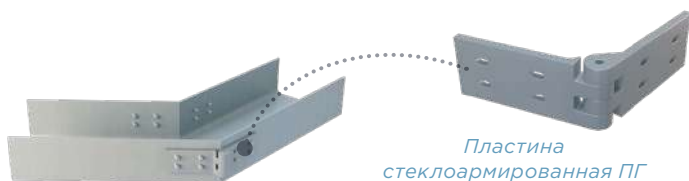
Рис. 44. Организация поворота кабельных лотков
