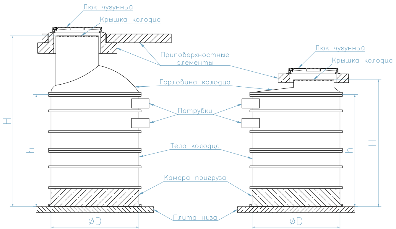
Колодец для установки под автодорогой
