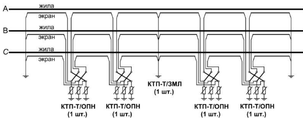
Рис. 25. Схема транспозиции экранов (два полных цикла)
