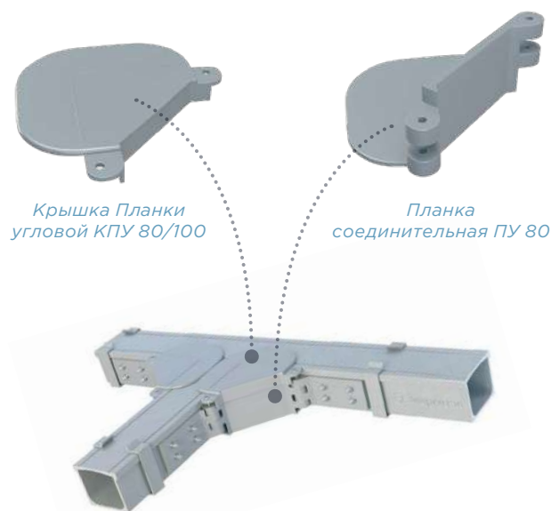
Рис. 45. Организация Т-образного ответвителя
