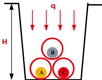
Рис. 54. Воздействие на трубу вертикальной нагрузки q (в качестве примера показан пучок из трех труб с кабелями фаз А, В, С)
