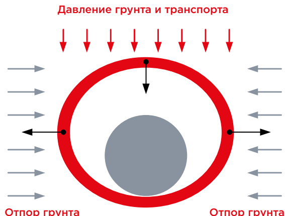
Рис. 55. Полимерная труба с кабелем под давлением грунта
