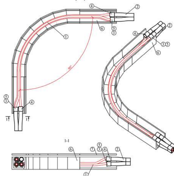
Исполнение 1. Поворот трассы КЛ в железобетонных лотках
