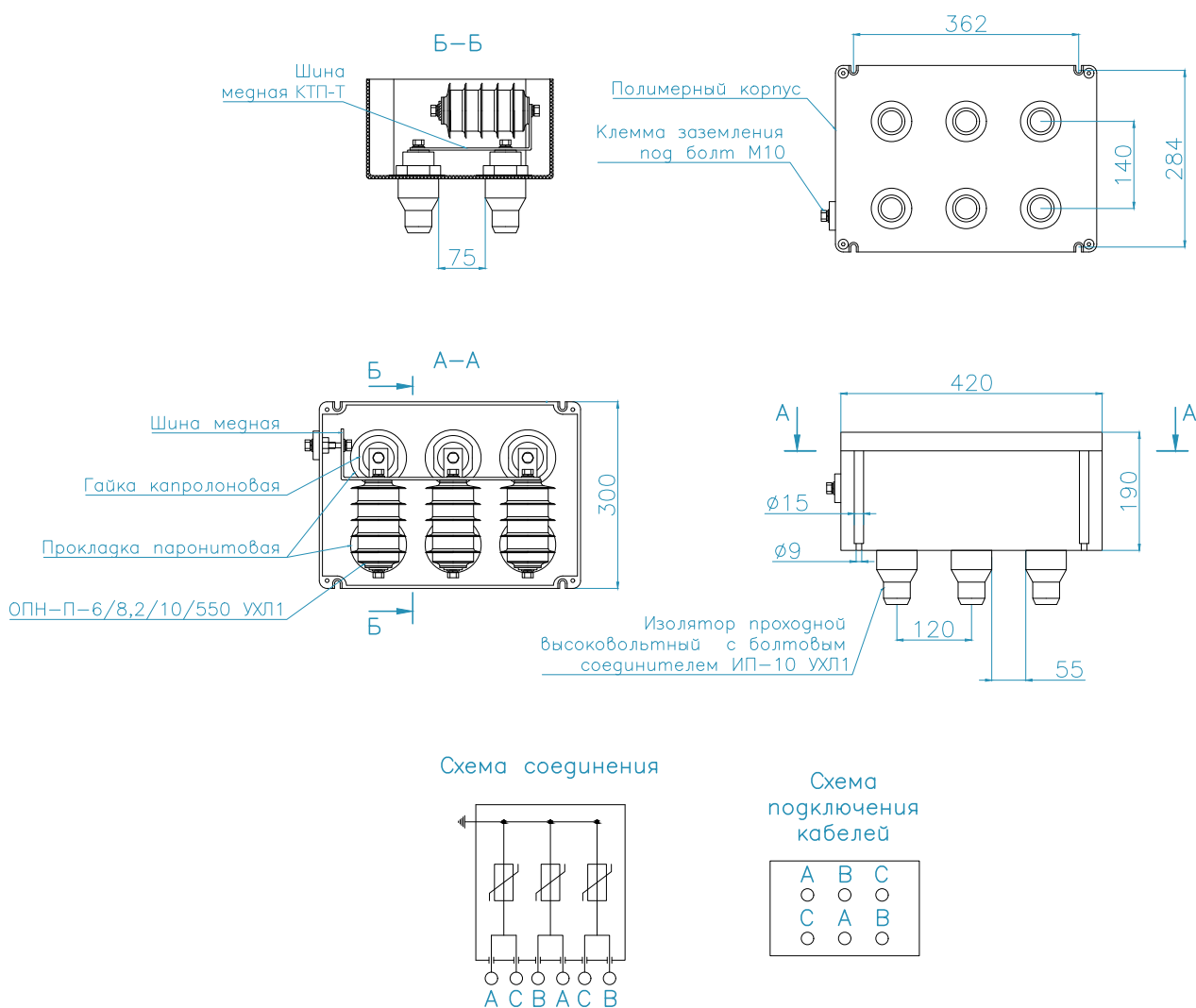
Рис. 24. Коробка транспозиции Энерготэк КТП-Т/ОПН-8,2-550
