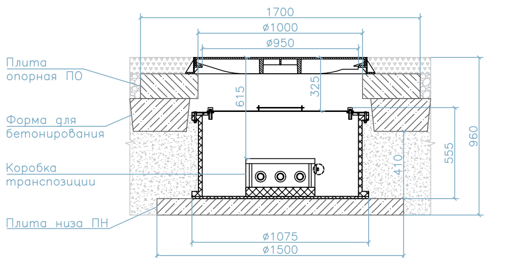
Чертежи узла транспозиции ПротекторФлекс® УТП 1000/500 1хКТП-ТС/ОПН-8,2-550
