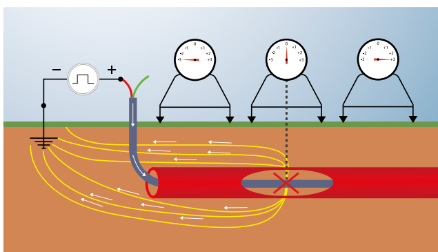
Рис. 3. Испытания оболочки кабеля в токопоисковых трубах ПротекторФлекс® ОМП. ОМП-труба не препятствует определению факта и места повреждения кабеля в трубе
