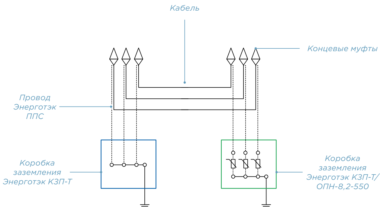
Рис. 28. Схема одностороннего заземления экранов кабелей с применением коробок заземления концевых Энерготэк
