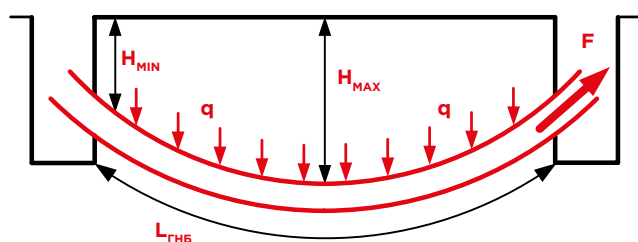
Рис. 57. Протяжка трубы в буровом канале
