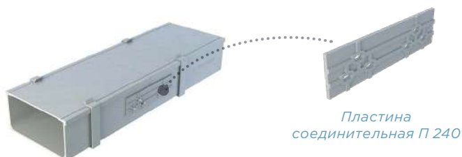
Рис. 42. Прямолинейное соединение кабельных лотков
