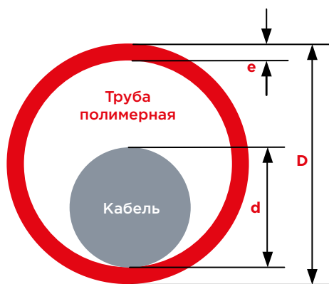
Рис. 56. Труба с проложенным в ней кабелем
