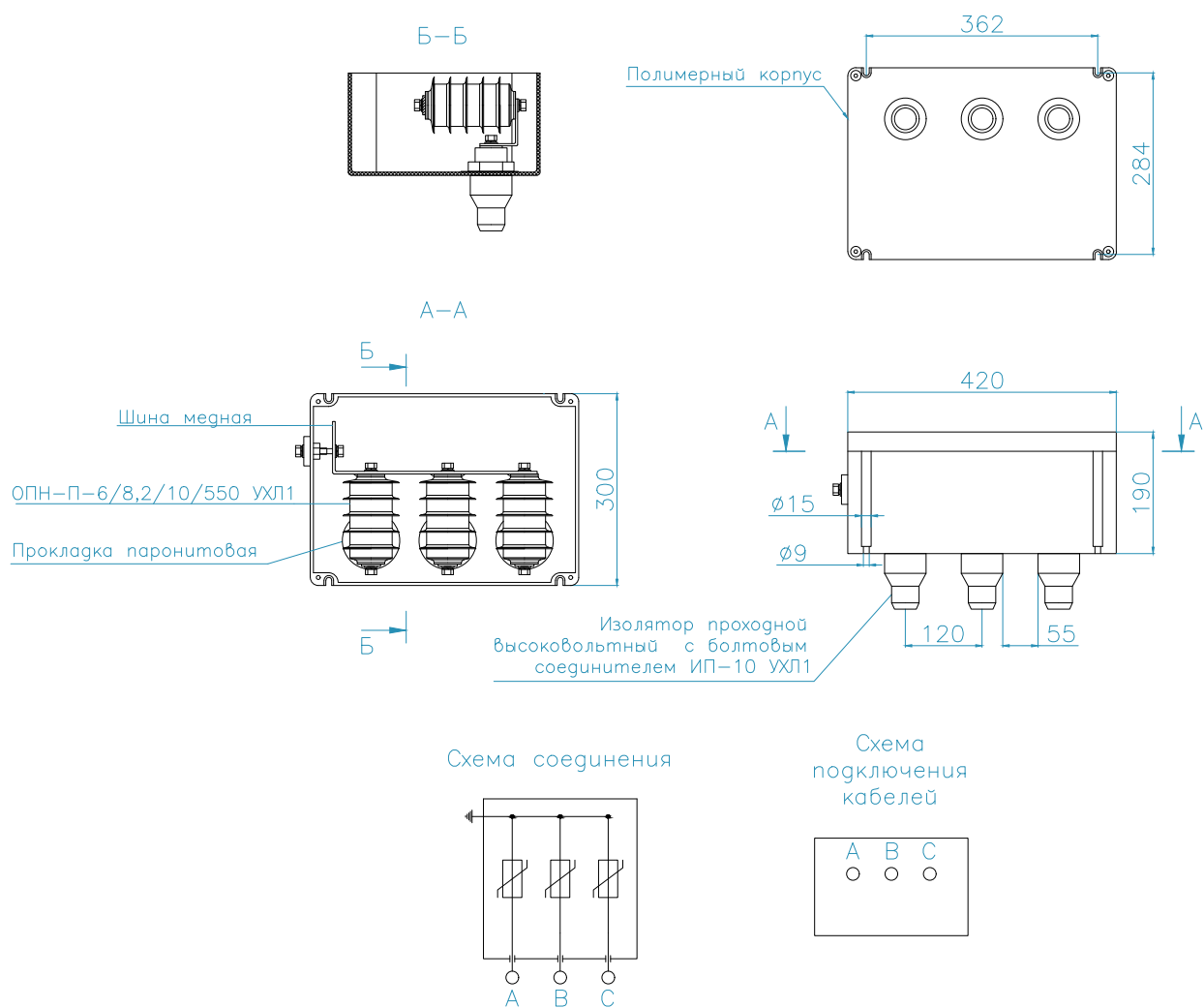
Рис. 30. Коробки заземления Энерготэк КЗП-Т IP68/ОПН-8,2-550 А
