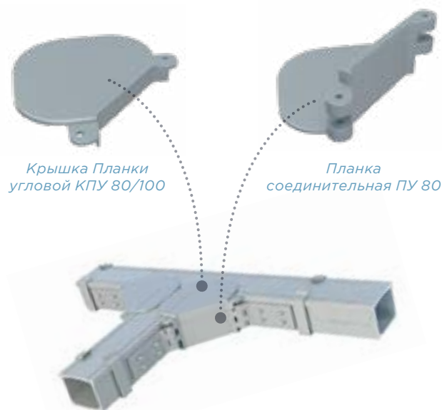
Рис. 50. Организация Т-образного ответвителя
