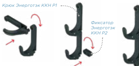
Рис. 57. Схема сборки крюков Энерготэк ККН
