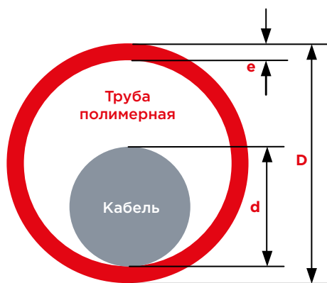
Рис. 59. Труба с проложенным в ней кабелем
