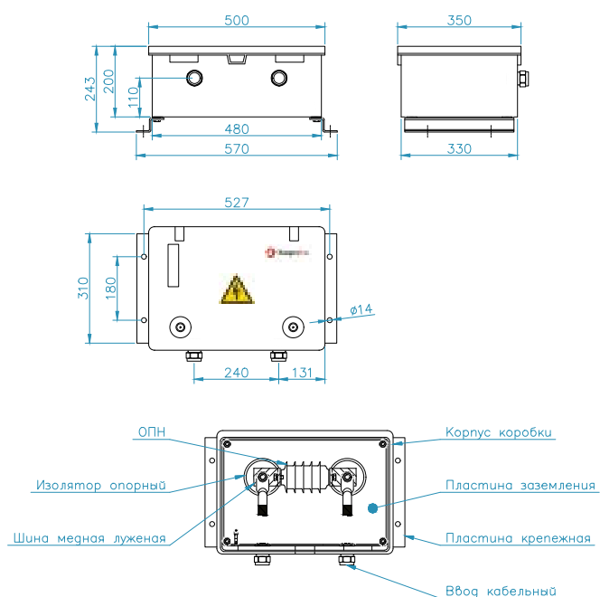
Рис. 35. Коробка заземления Энерготэк КЗП-О/ОПН-8,2-550
